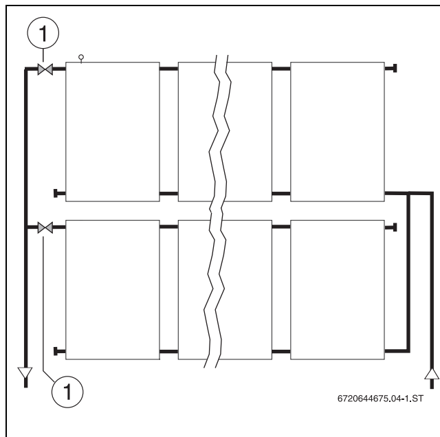
Рис. 27 Промывка параллельно включенных коллекторных полей
