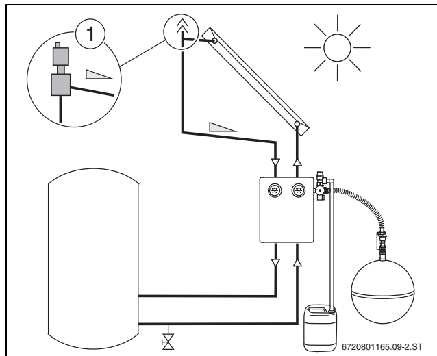
Рис. 11 Положение автоматического воздушного клапана
