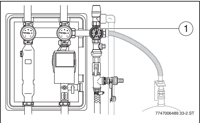
Рис. 33 Контроль стрелки манометра
