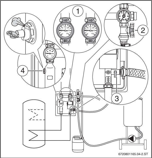
Рис. 32 Закрытие и открытие кранов для наполнения и слива
