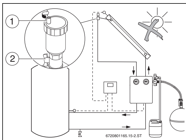
Рис. 40 Закрыть запорный винт воздухоотделителя и шаровой кран
