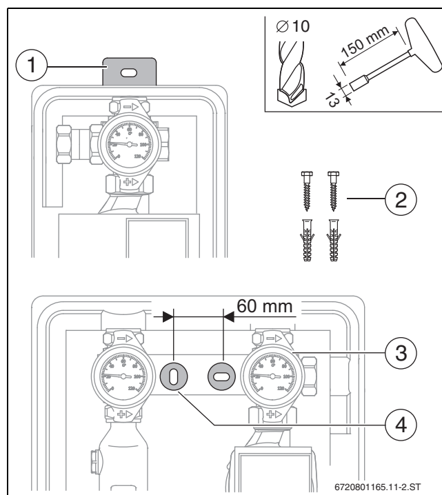
Рис. 15 Монтаж станции
