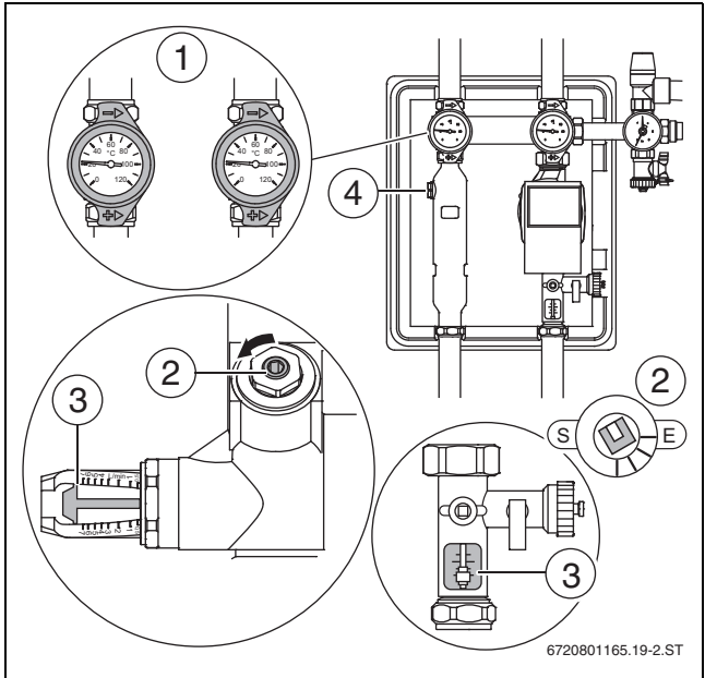
Рис. 41 [1] Гравитационные тормоза в работоспособном состоянии [2] Регулировочный винт на ограничителе потока, зависит от исполнения [3] Указатель объёмного потока, зависит от исполнения [4] Удаление воздуха на воздухоотделителе
