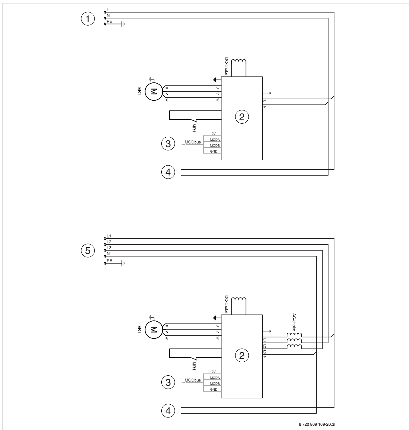
Рис. 20 Электропитание преобразователя
