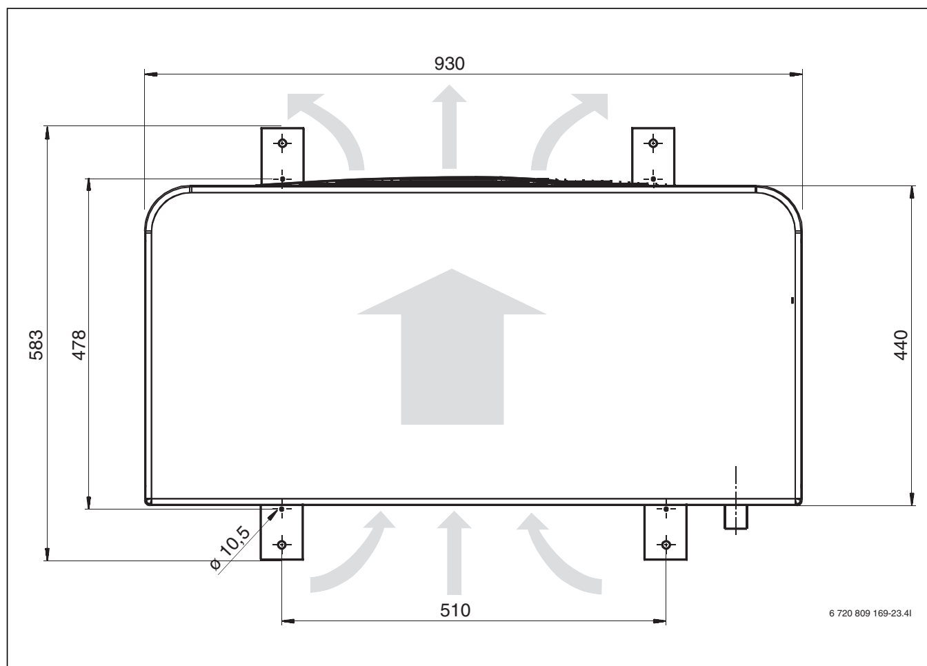
Рис. 6 Размеры тепловых насосов типов 5, 7, 9, вид спереди
