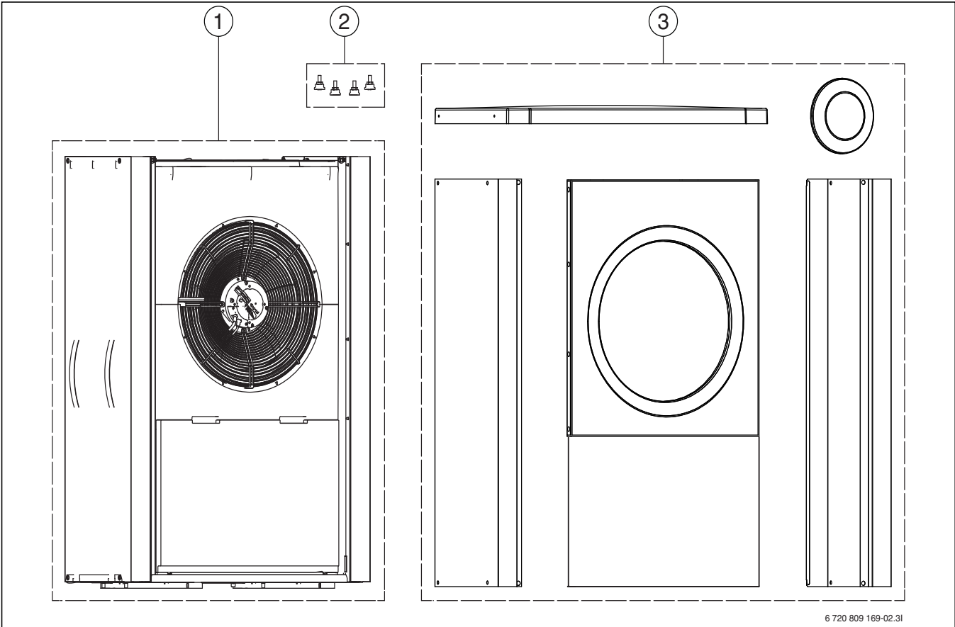
Рис. 1 Комплект поставки
