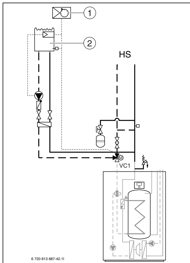
Рис. 33 Пример отопительной системы с бассейном
