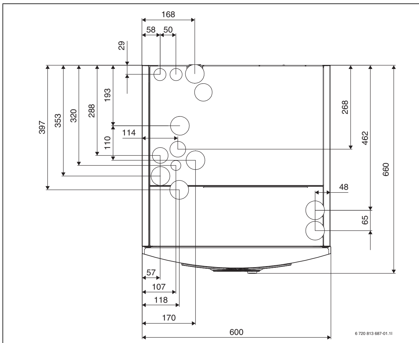
Рис. 8 Подсоединительные размеры, вид сверху
