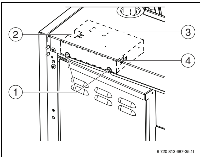
Рис. 35 Монтаж и подключение IP-модуля
