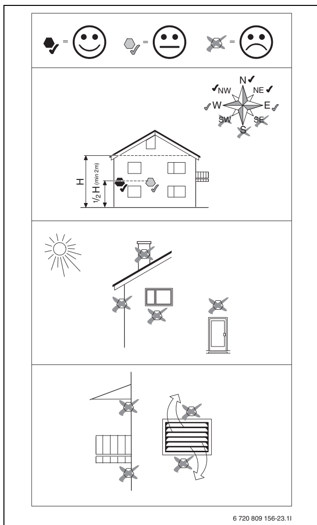
Рис. 25 Установка датчика наружной температуры
