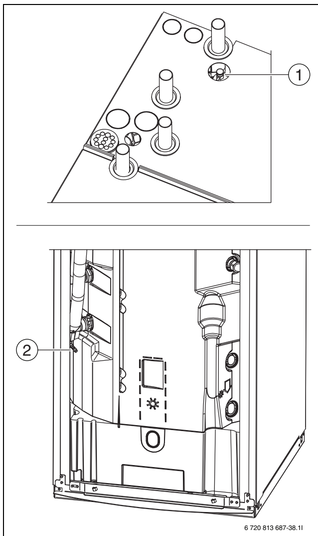
Рис. 21 Точки удаления воздуха
