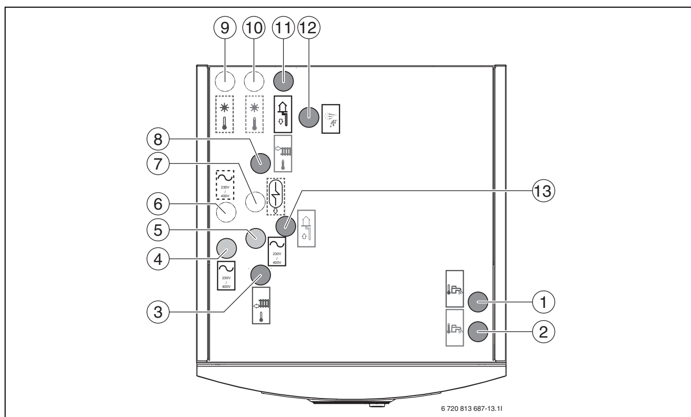
Рис. 9 Подключения теплового насоса
