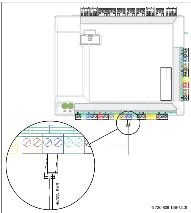
Рис. 32 EMS-подключение к монтажному модулю
