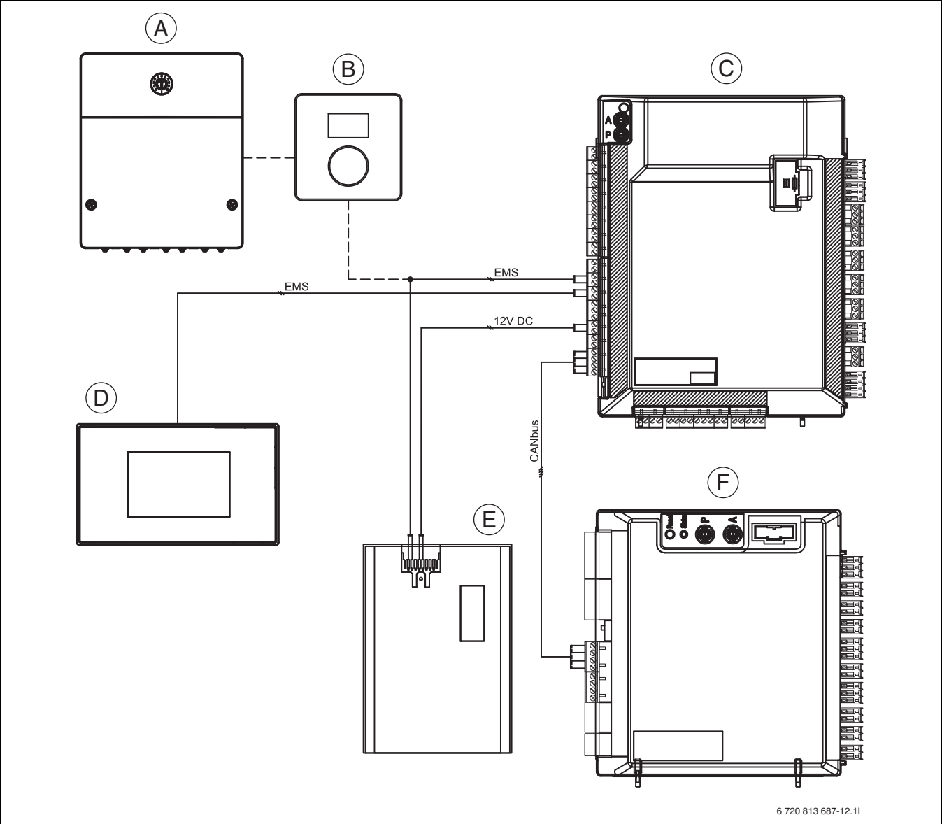
Рис. 31 Обзор CAN-BUS и EMS
