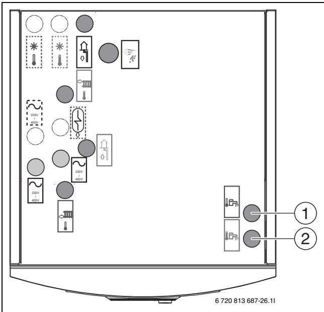
Рис. 22 Подключения воды к теплому насосу
