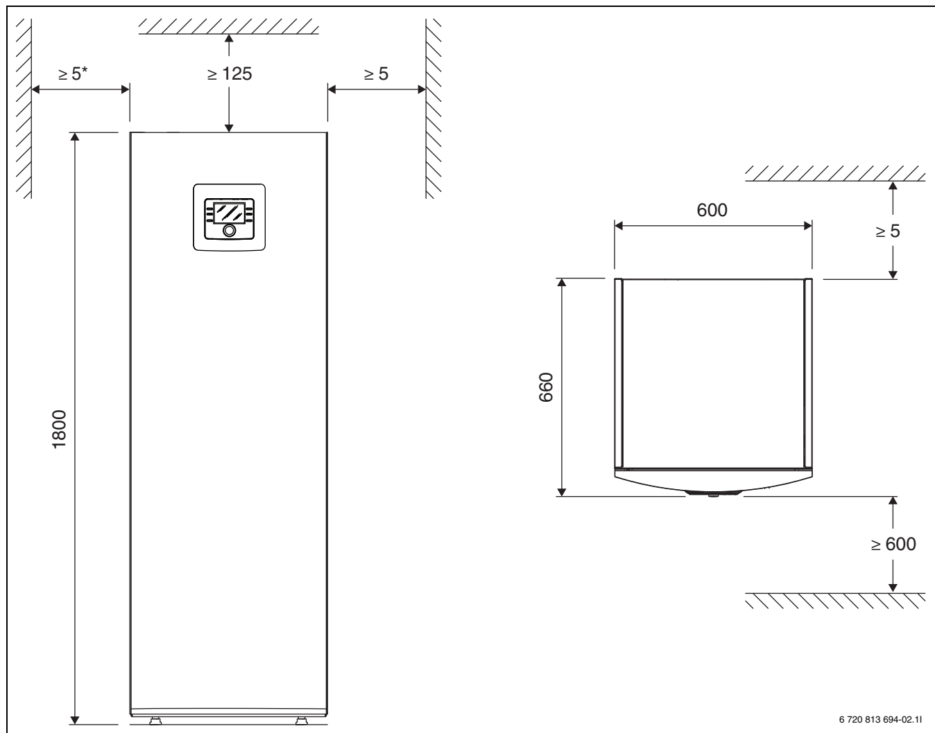
Рис. 7 Размеры и рекомендуемые минимальные расстояния, вид спереди и сверху
