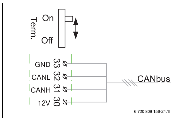
Рис. 23 Терминирование CAN-BUS
