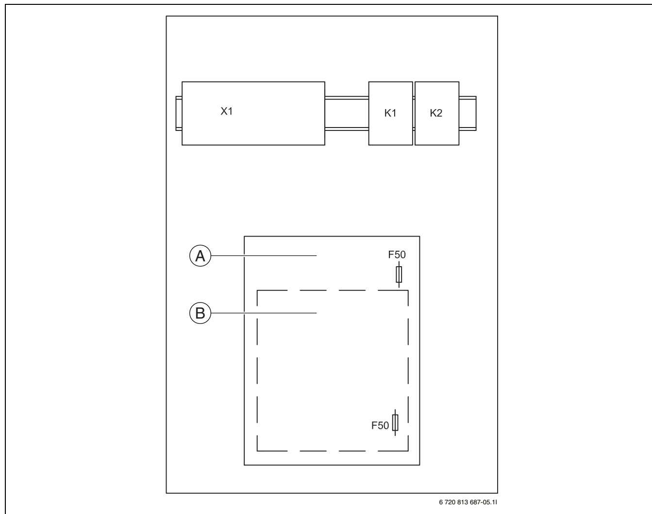
Рис. 26 Расположение в распределительной коробке
