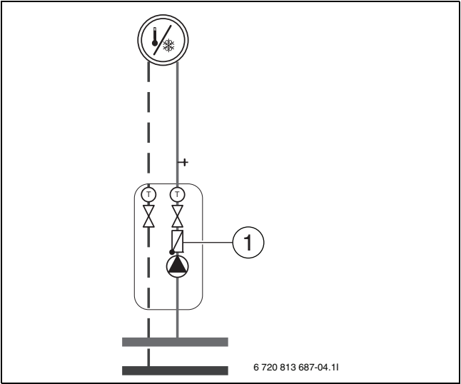
Рис. 4 Отопительный контур
