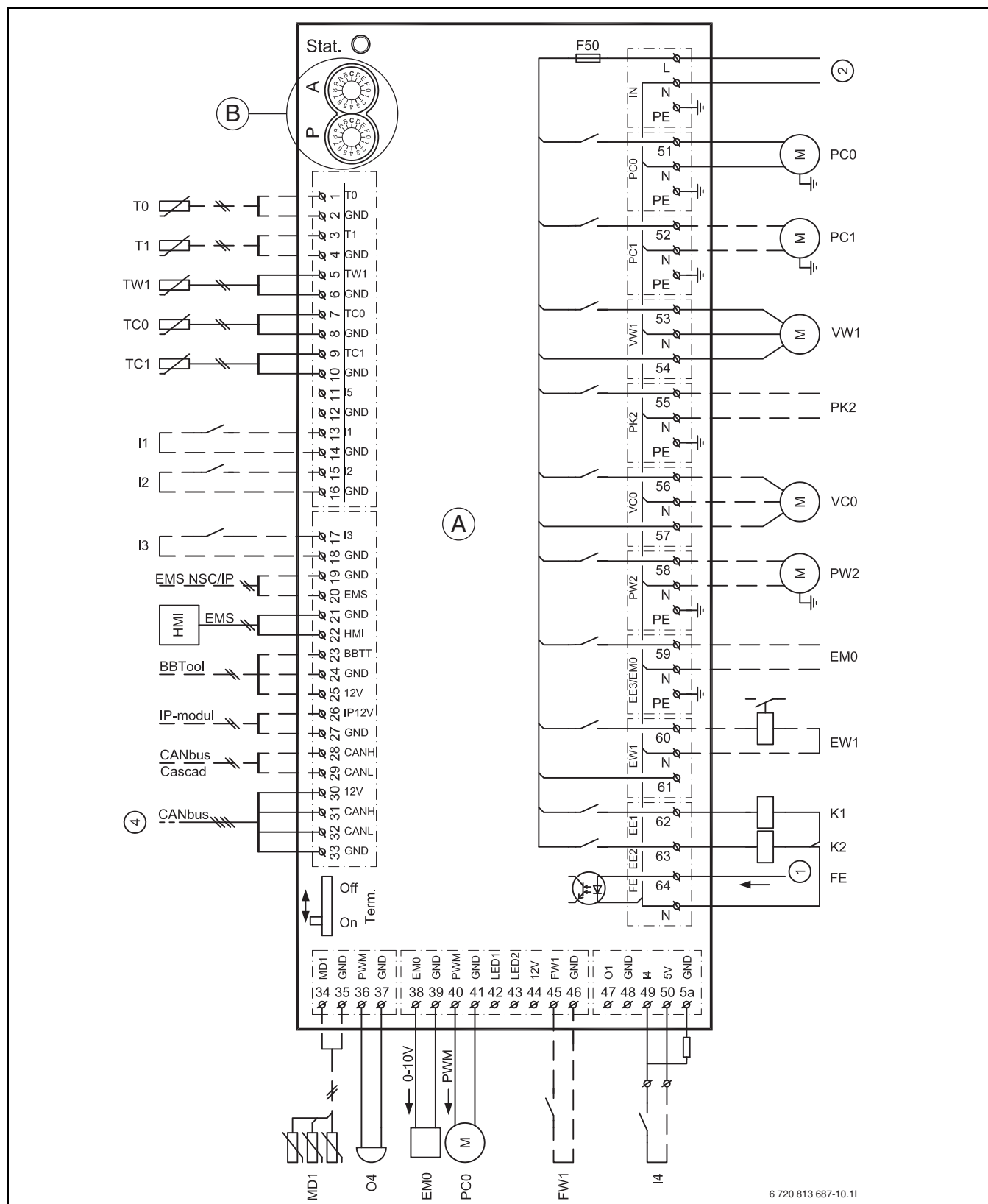
Рис. 29 Электросхема, монтажный модуль
