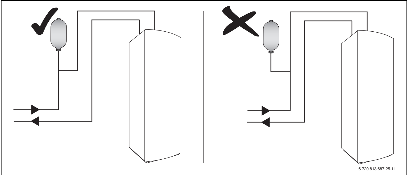
Рис. 11 Монтаж расширительного бака
