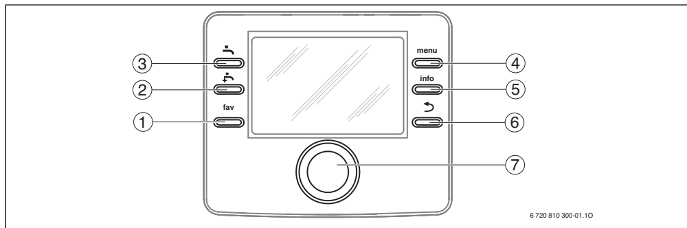
Рис. 1 Элементы управления
