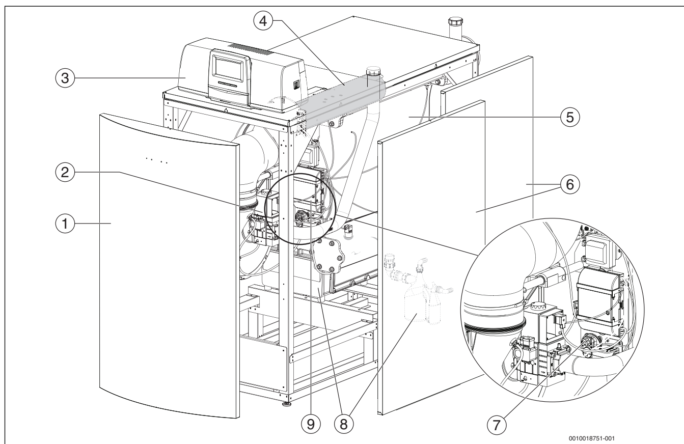
Рис. 1 Logano plus GB402, 395...620 кВт—основные составные части
