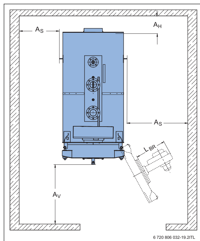
Рис. 13 Помещение для установки котла (размеры в мм)
