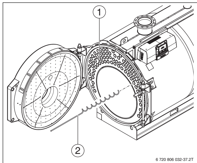
Рис. 29 Удаление турбуляторов
