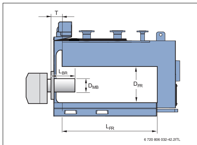
Рис. 4 Размеры двери горелки и горелки SK655/SK755 2)
