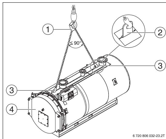
Рис. 12 Подъём котла краном
