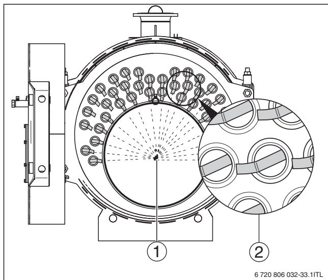
Рис. 33 Установка турбуляторов
