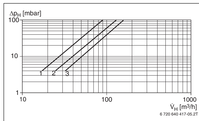
Рис. 9 Падение давления на стороне воды Logano SK755
