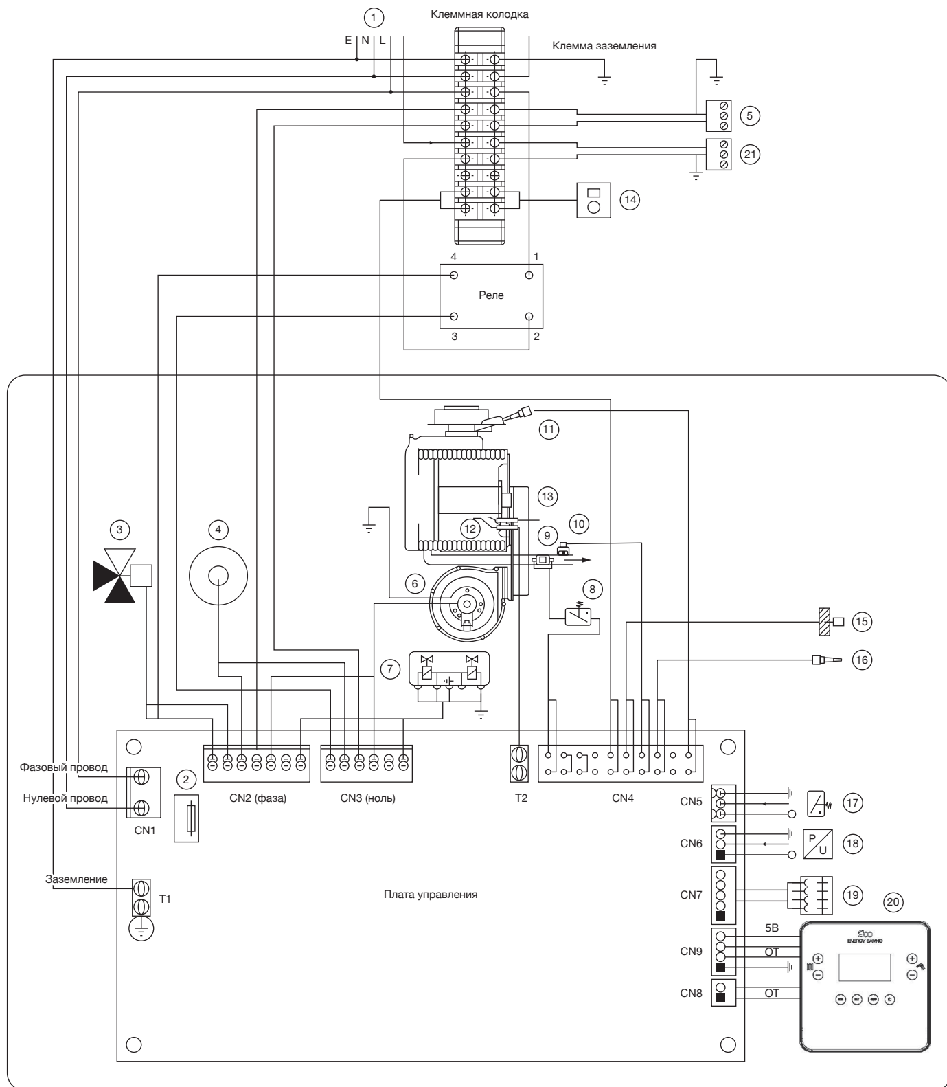
Рис. 38. Электрическая схема платы.
