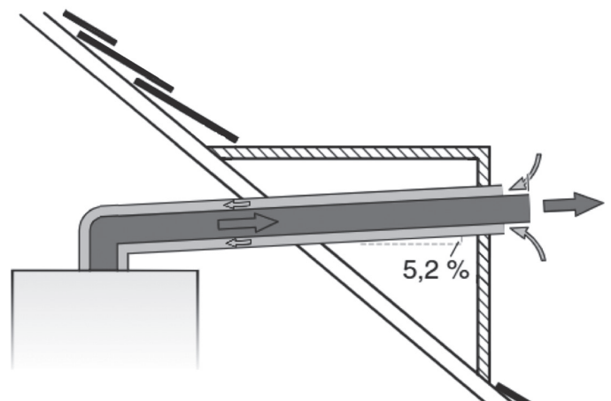
Рис. 36. Угол наклона дымохода.
