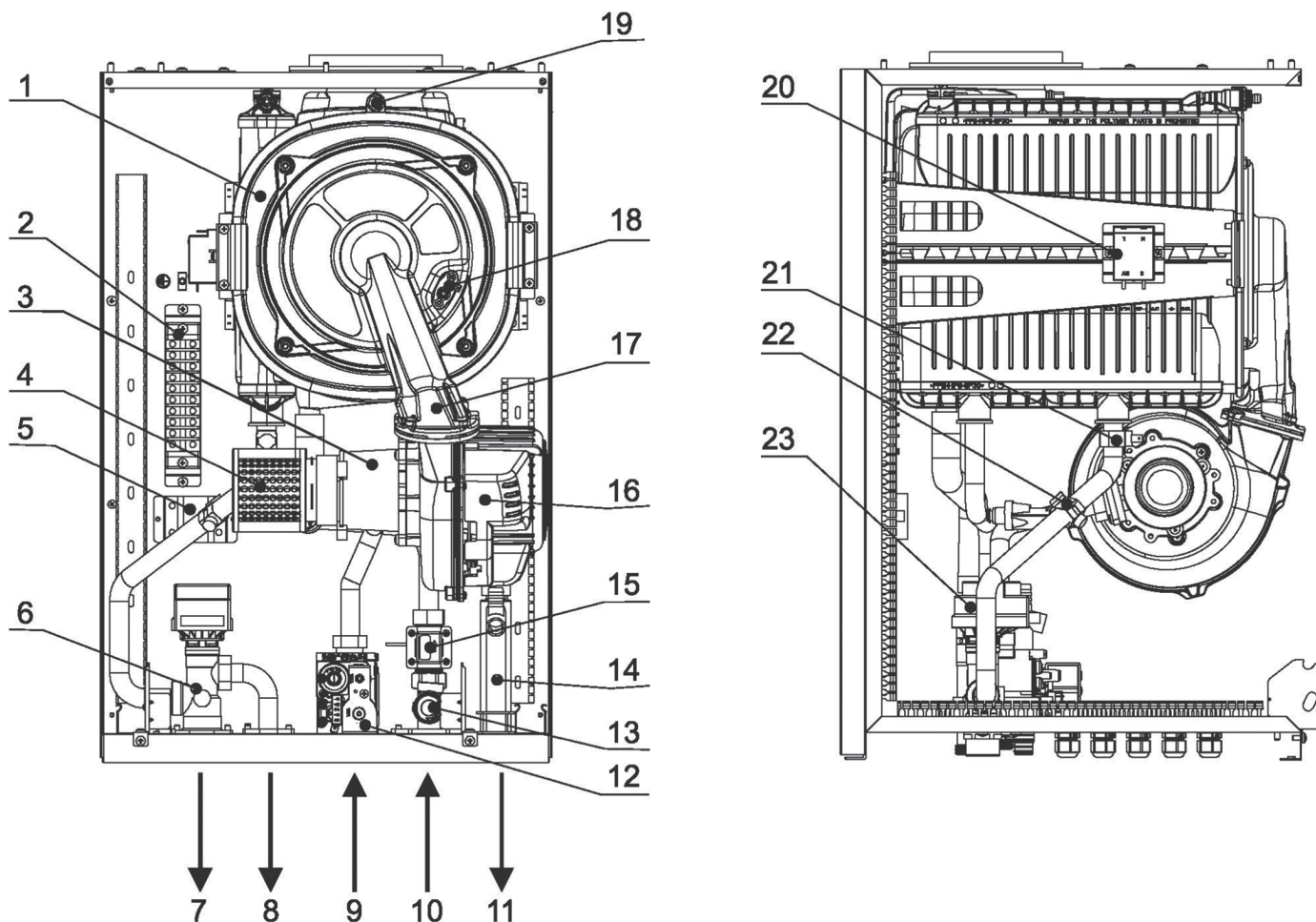
Рис. 2. Общая схема.
