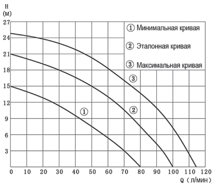
Рис. 39. Рекомендуемые характеристики котлового насоса.
