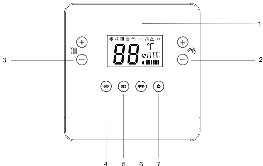
Рис. 8. Панель управления.
