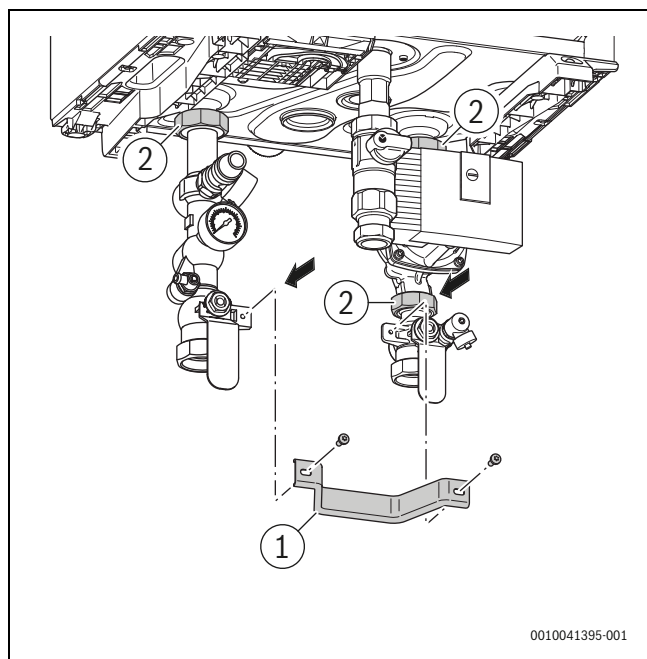
Рис. 15 Монтаж скоб
