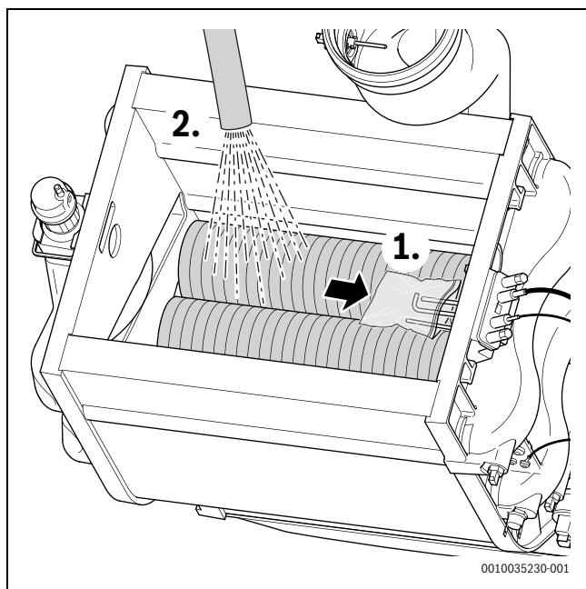
Рис. 43 Чистка теплообменника
