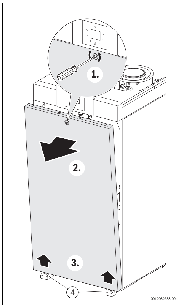
Рис. 6 Открытие передней стенки
