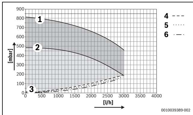
Рис. 51 Остаточный напор насоса GB272-50
