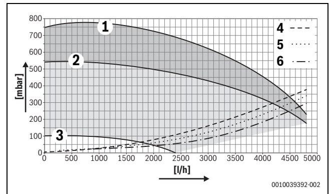
Рис. 54 Остаточный напор насоса GB272-100
