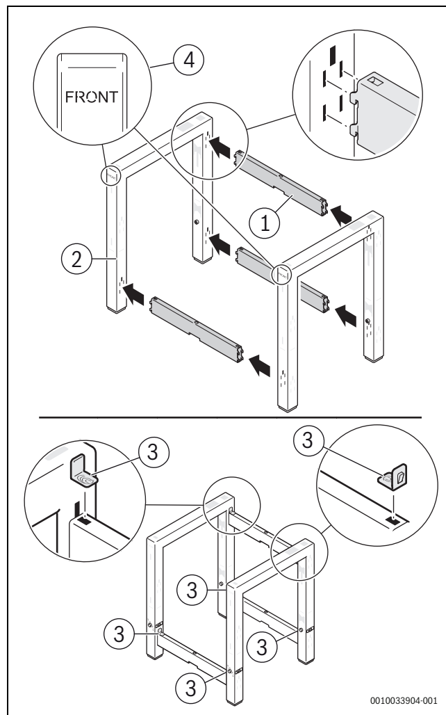
Рис. 8 Установка рамы
