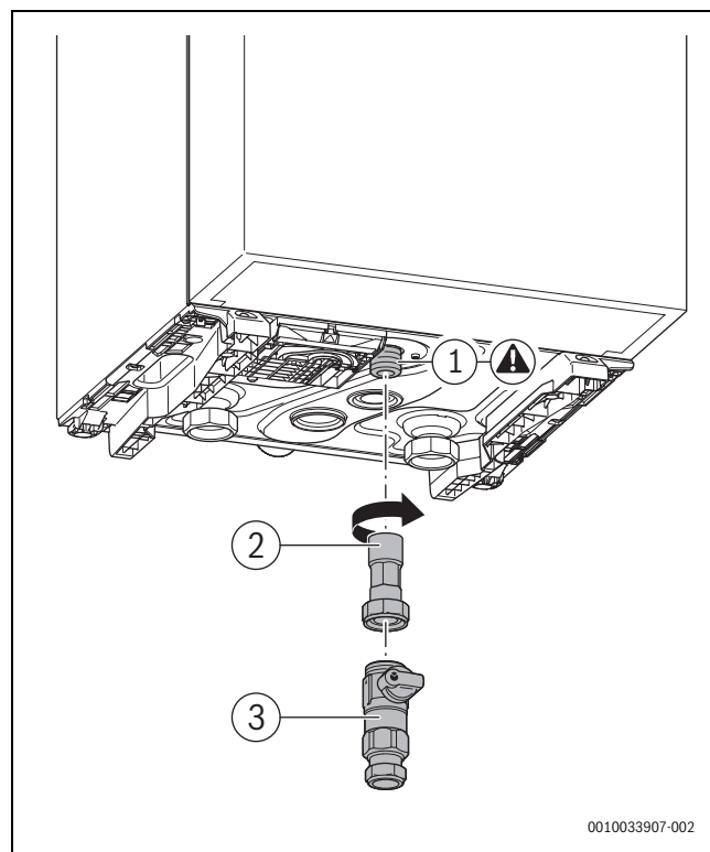
Рис. 13 Установка газового клапана
