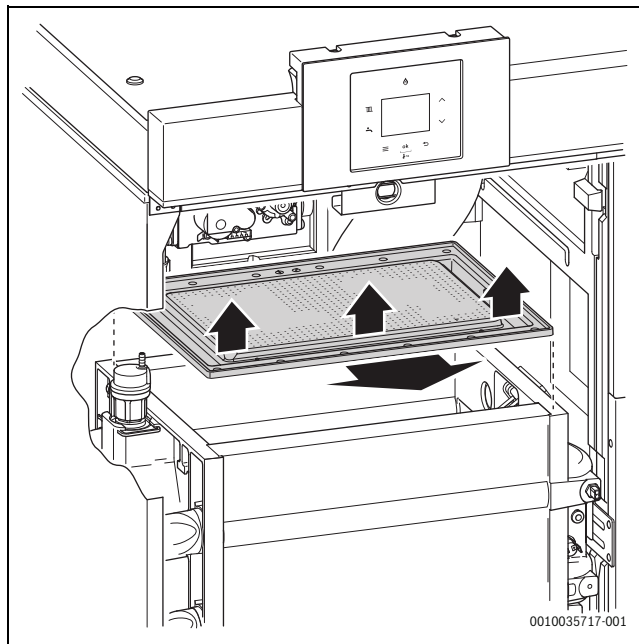
Рис. 42 Снятие горелки
