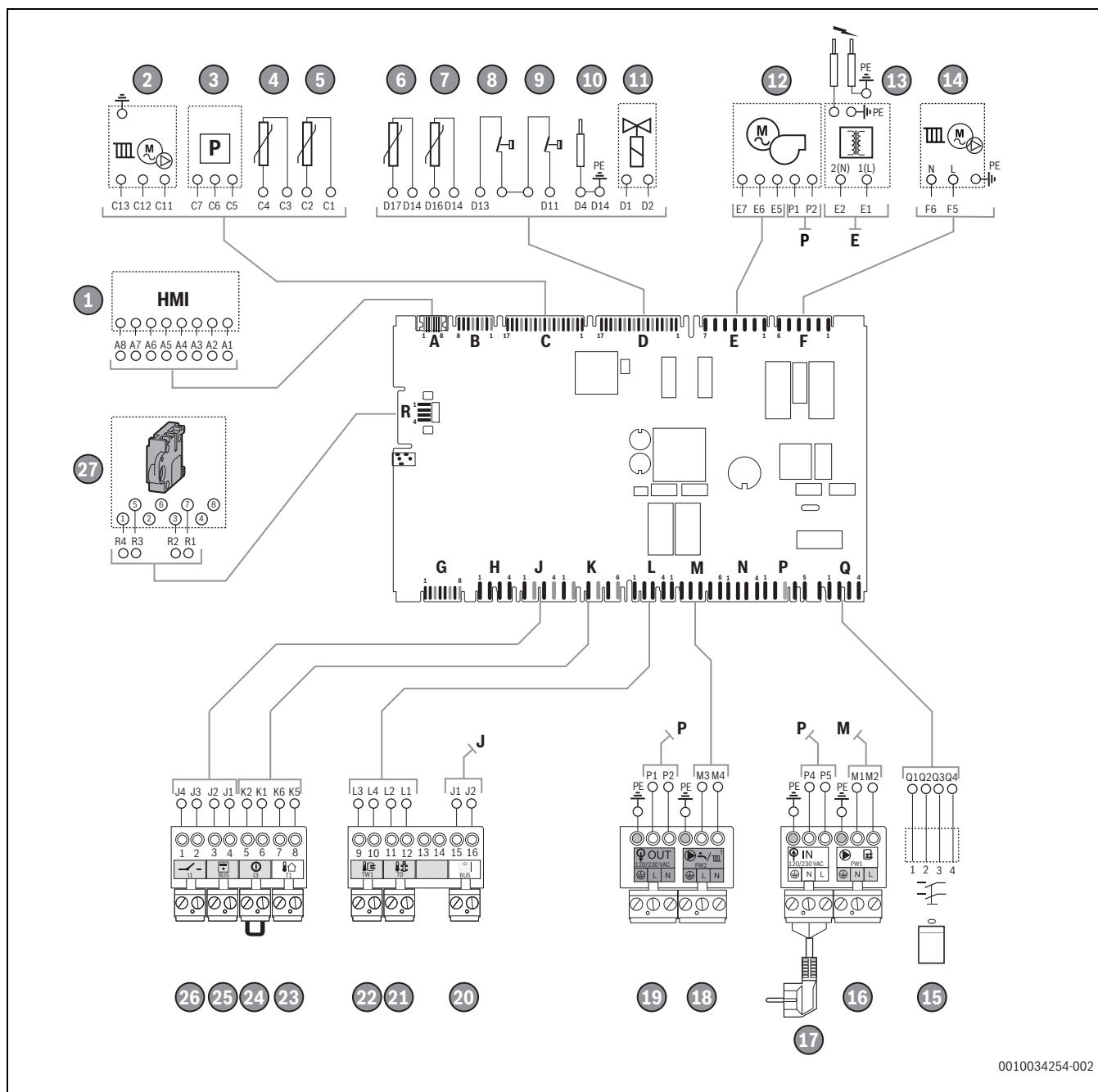
Рис. 50 Электрическая схема
