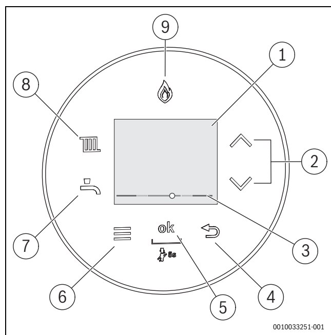
Рис. 36 Панель управления
