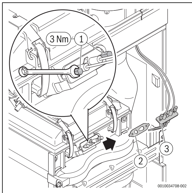
Рис. 47 Установка запальника
