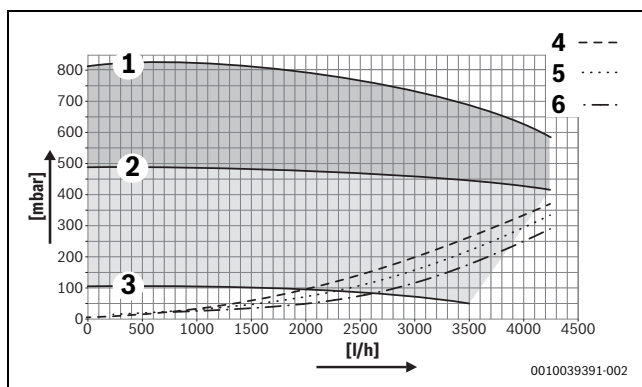
Рис. 53 Остаточный напор насоса GB272-85
