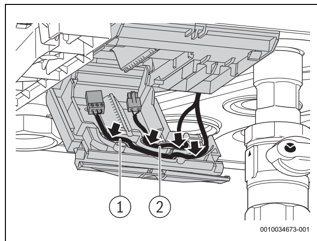
Рис. 26 Подключение насоса
