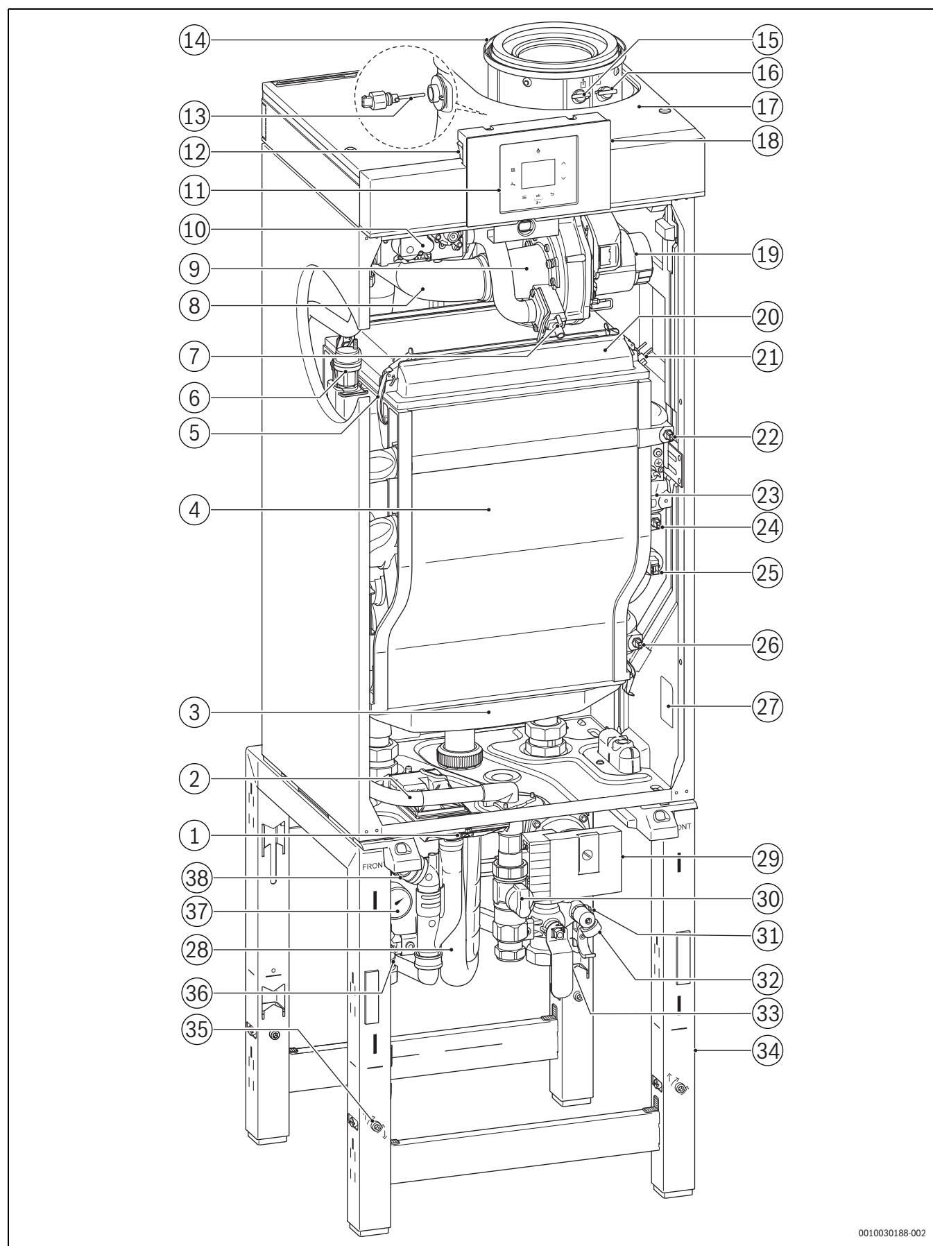
Рис. 1 GB272 с комплектом подсоединения на раме
