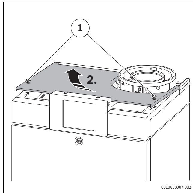
Рис. 22 Открытие крышки
