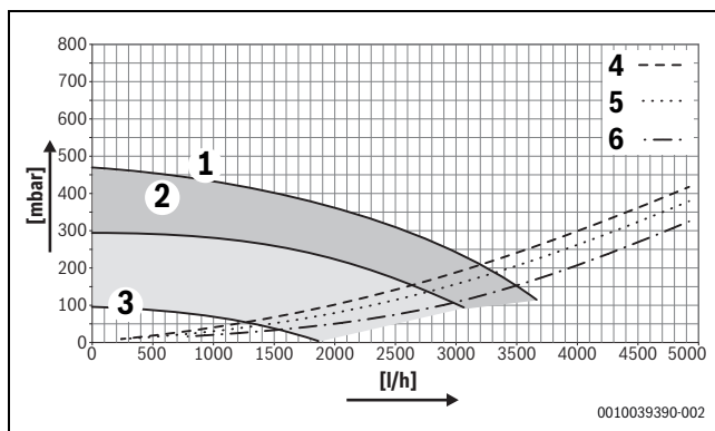
Рис. 52 Остаточный напор насоса GB272-70
