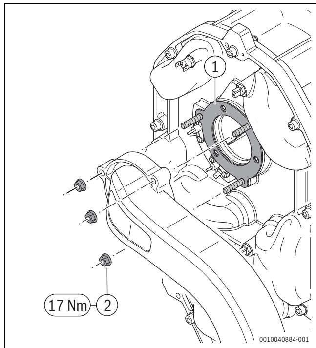
Рис. 44 Установка трубы для смешивания газа и воздуха
