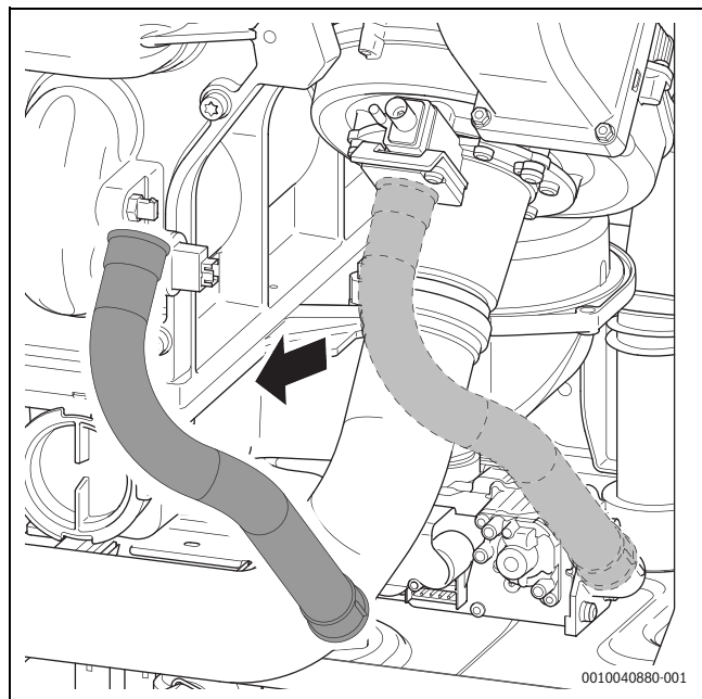
Рис. 36 Отсоединение газового шланга
