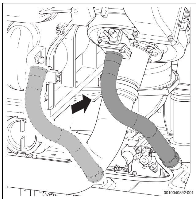
Рис. 46 Установка газового шланга
