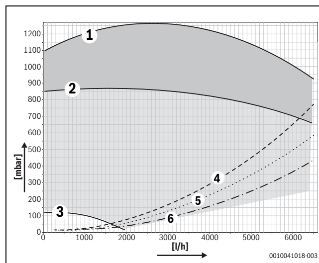
Рис. 51 Остаточный напор насоса GB272-125, GB272-150
