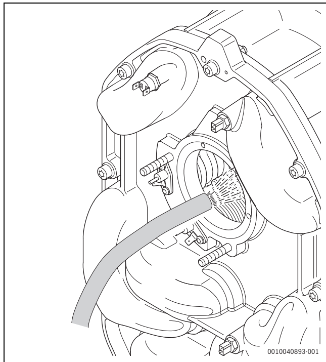
Рис. 40 Промывка теплообменника
