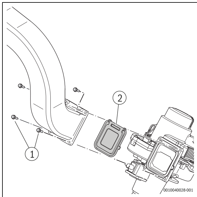
Рис. 48 Замена обратного клапана для отвода дымовых газов
