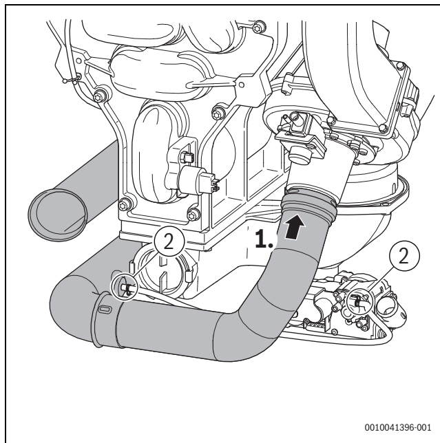
Рис. 45 Проверьте соединения шланга для компенсации давления
