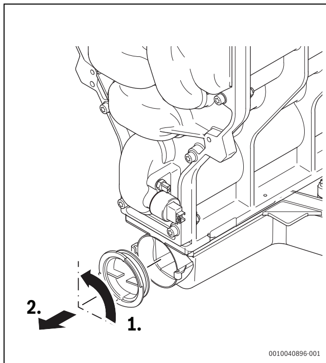
Рис. 41 Откройте крышку конденсатной ванны.
