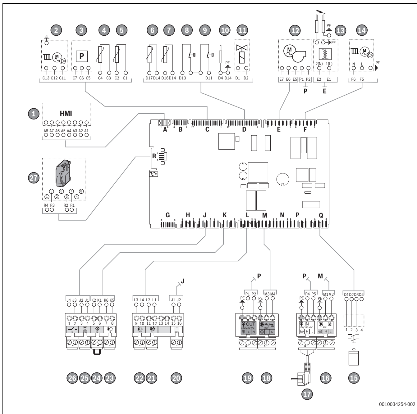
Рис. 50 Электрическая схема
