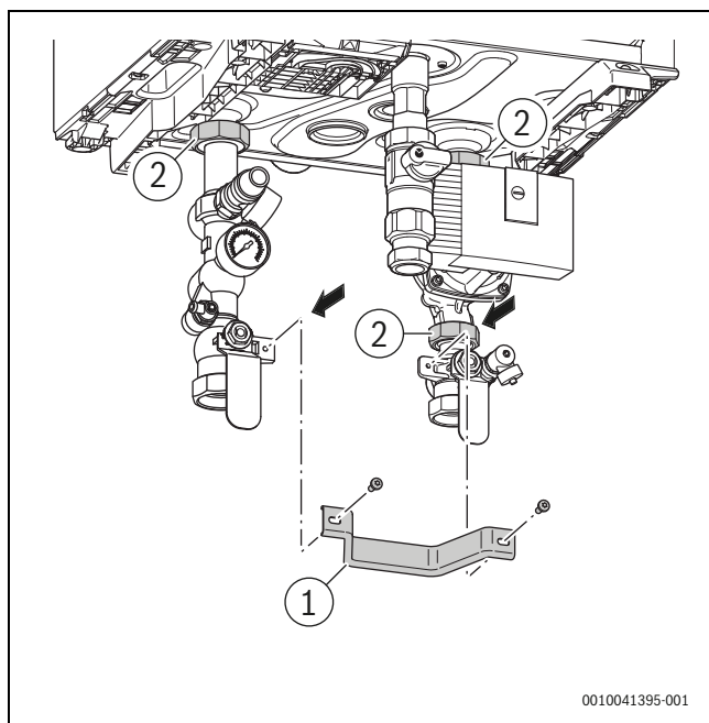
Рис. 15 Монтаж скоб
