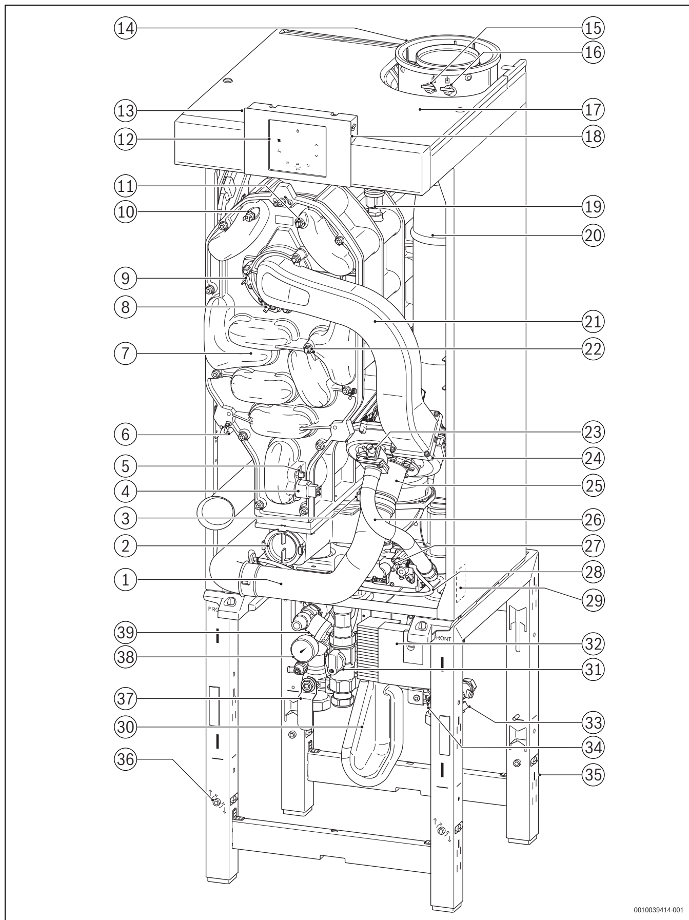
Рис. 1 GB272 с комплектом подключения на раме
