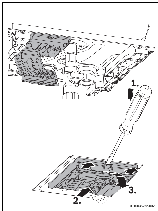
Рис. 25 Открытие клеммного блока насоса
