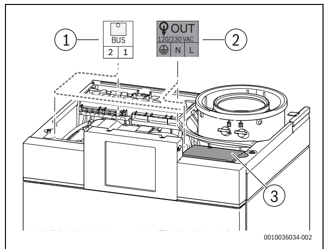
Рис. 29 Монтаж функционального модуля
