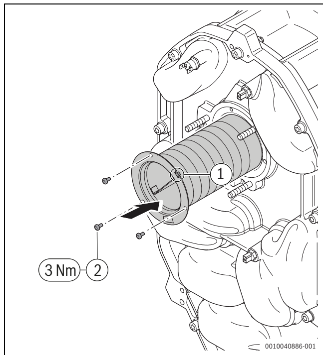
Рис. 43 Установка горелки
