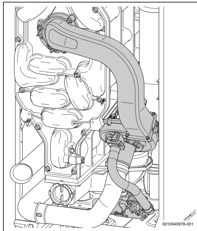
Рис. 34 Контрольные осмотры газовой раппы
