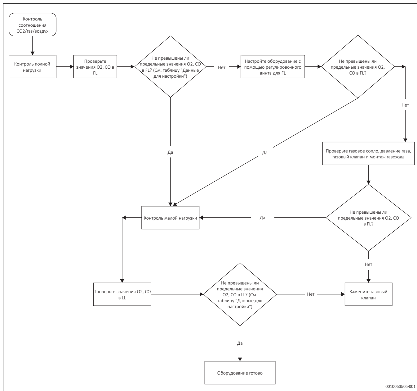
Рис. 33 Технологическая схема с инструкциями по регулировке
