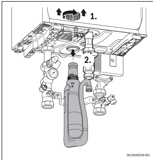
Рис. 42 Демонтаж сифона котла
