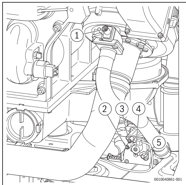
Рис. 31 Обзор штуцеров для выполнения замеров регулировочных винтов
