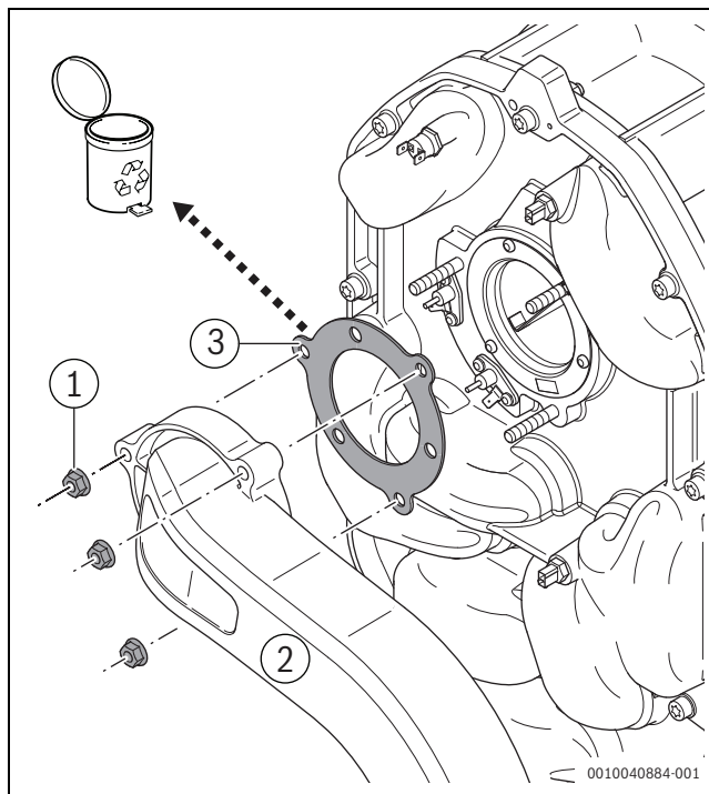
Рис. 38 Демонтаж трубы для смешивания газа и воздуха
