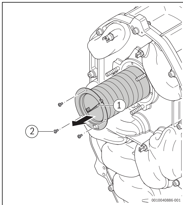
Рис. 39 Разборка горелки
