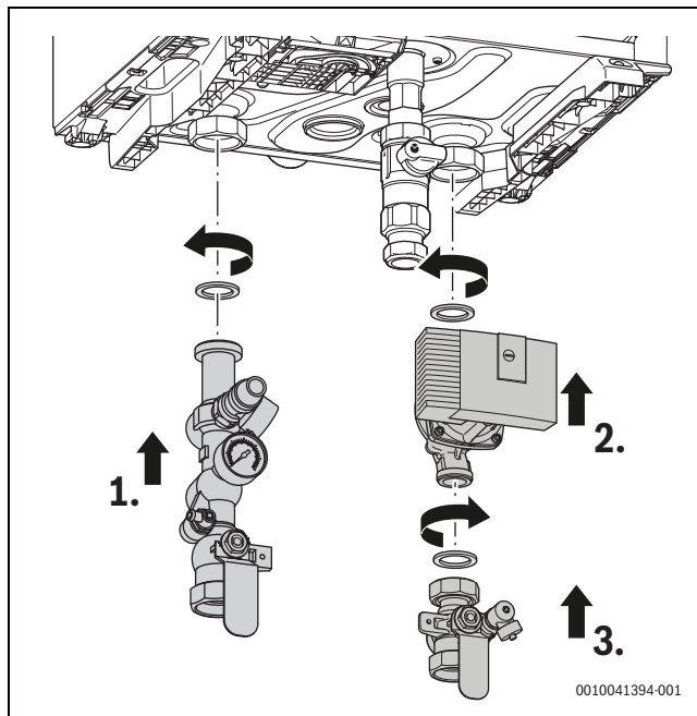
Рис. 14 Монтаж подключения подающей/обратной линии
