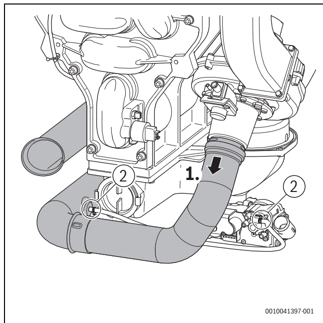
Рис. 37 Демонтаж воздушного коллектора
