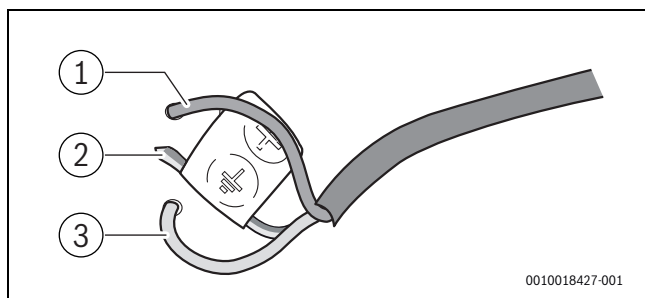
Рис. 30 Установка штекера
