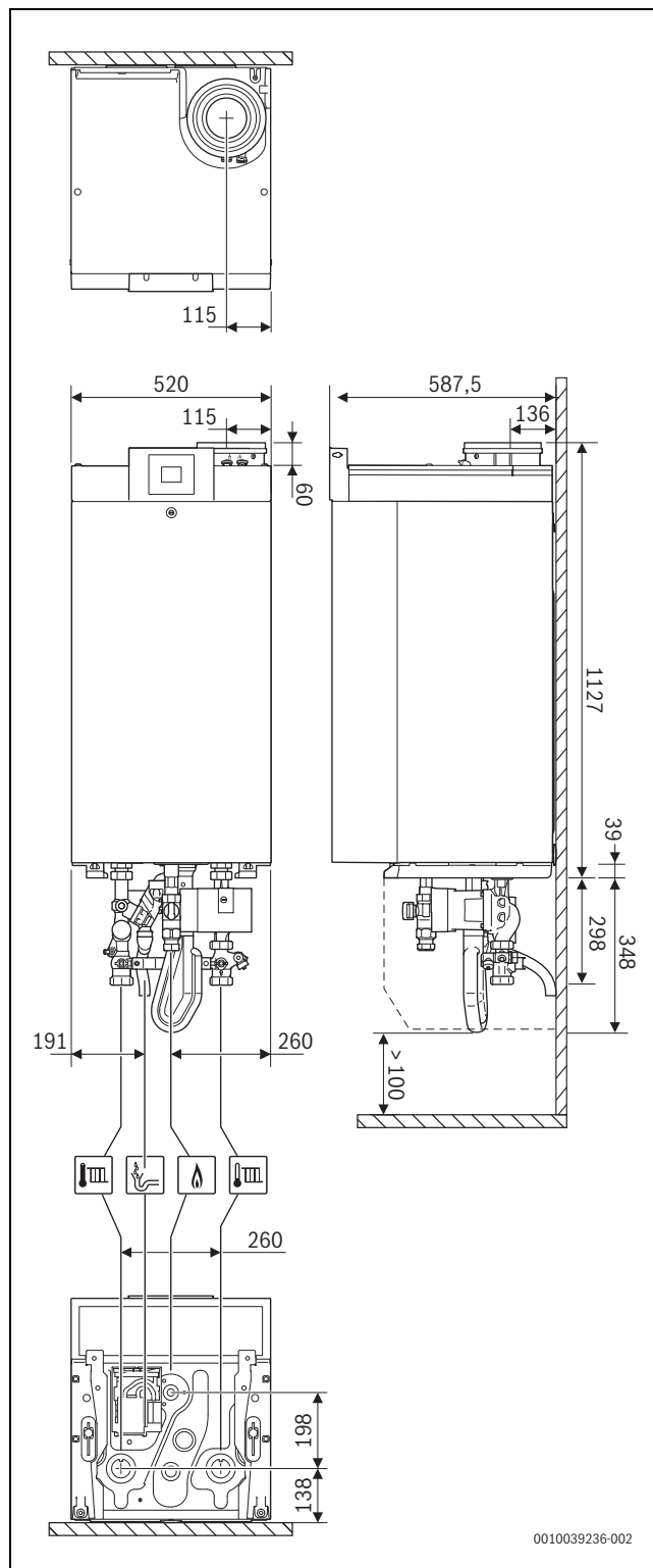
Рис. 3 Размеры на стене [мм]
