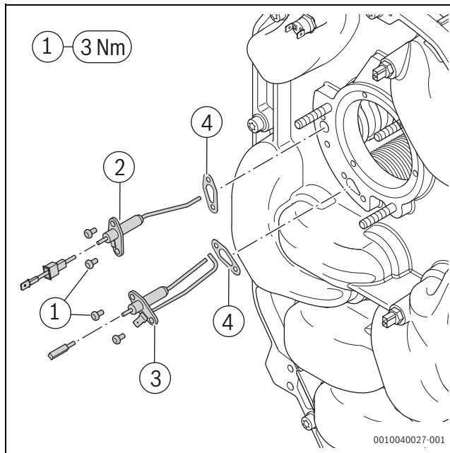
Рис. 47 Замена запального электрода ионизации
