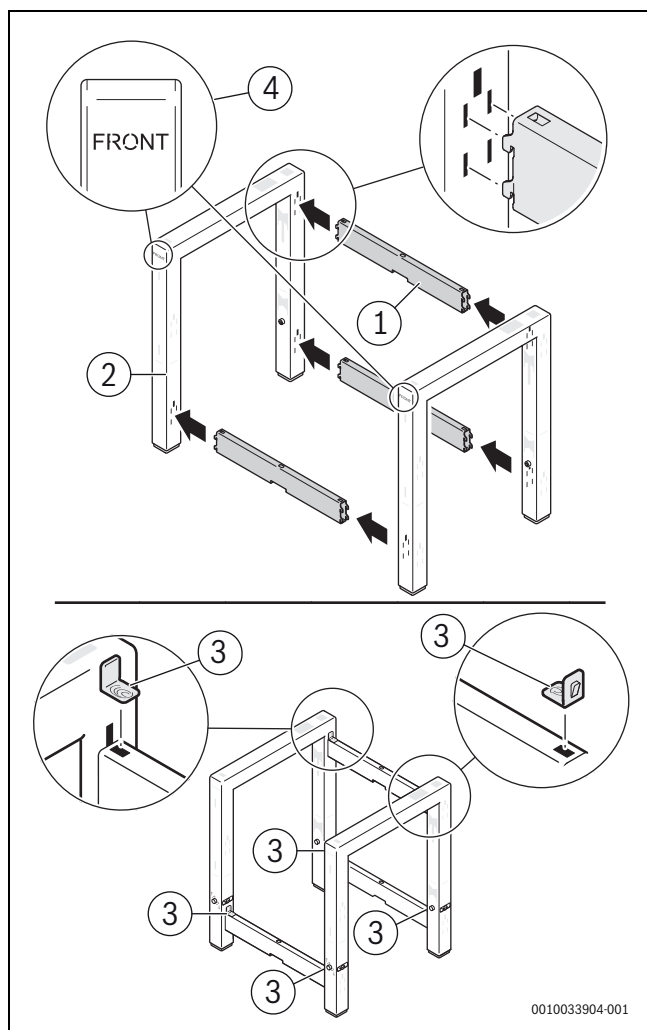
Рис. 8 Установка рамы
