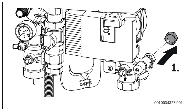
Рис. 20 Подключение расширительного бака
