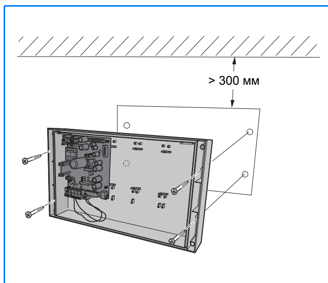
51/1 Необходимое свободное пространство над Easycom PRO
