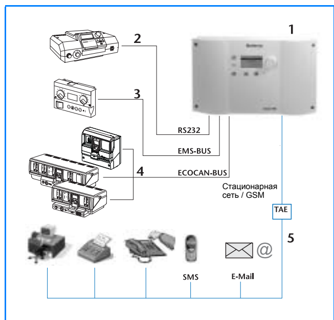
15/2 Варианты подключения к модему дистанционной связи Logamatic Easyscom PRO
