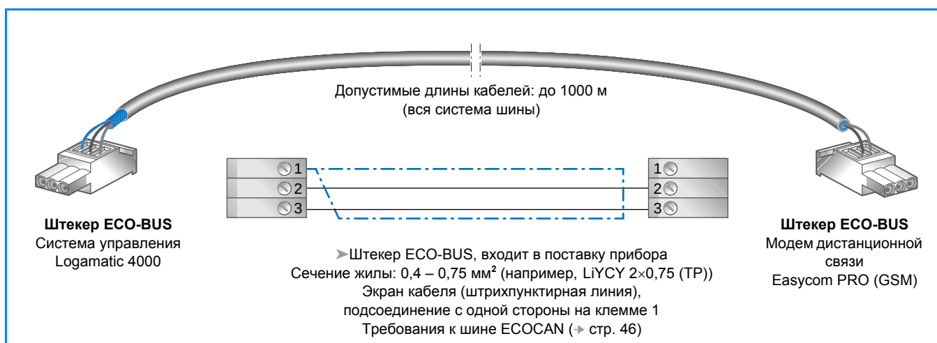
53/1 Разводка контактов соединительного кабеля шины ECOCAN между цифровой системой управления серии Logamatic 4000 и модемом дистанционной связи Easyscom PRO (GSM)
