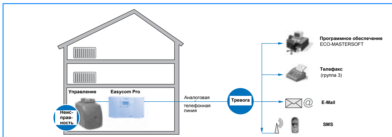
3/2 Установка с модемом дистанционной связи Logamatic Easycom или Easycom PRO: рабочие сообщения и сообщения о неисправностях передаются на один или несколько абонентов. Описание модема дистанционной связи → стр. 8.
