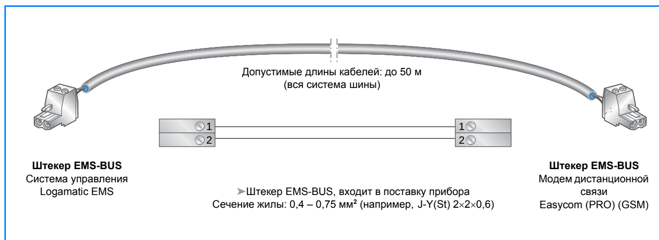
54/1 Разводка контактов для соединительного кабеля шины EMS между цифровой системой управления Logamatic EMS и модемом дистанционной связи Easycom (PRO) (GSM)
