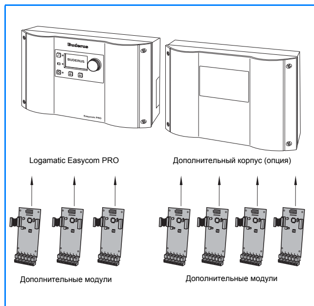
16/1 Easyscom PRO базовый прибор (слева) с 3 свободными разъемами и дополнительным корпусом (справа) с 4 свободными разъемами для модулей
